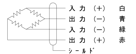
ケーブルの電氣的配線
